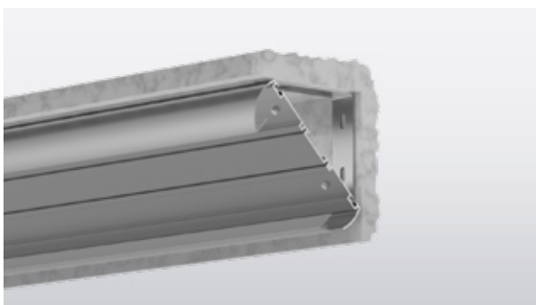
➤ Montagewinkel (Eckmontage) für Medienkanal 285 OVAL, Artikelnr. 620 104
