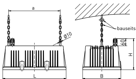
> POLARIS vorbereitet für Pendelabhängung Pendelabhängung und Deckenbefestigung sind bauseits zu liefern
